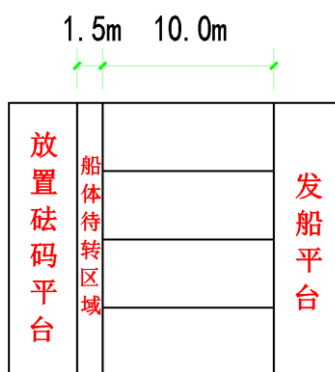
图3 运输赛场地示意图
