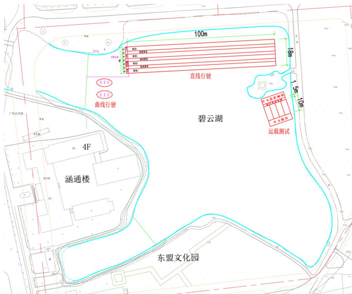
图5 直线竞速赛场地示意图
