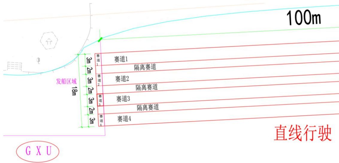
图6 直线竞速赛场地示细部示意图
